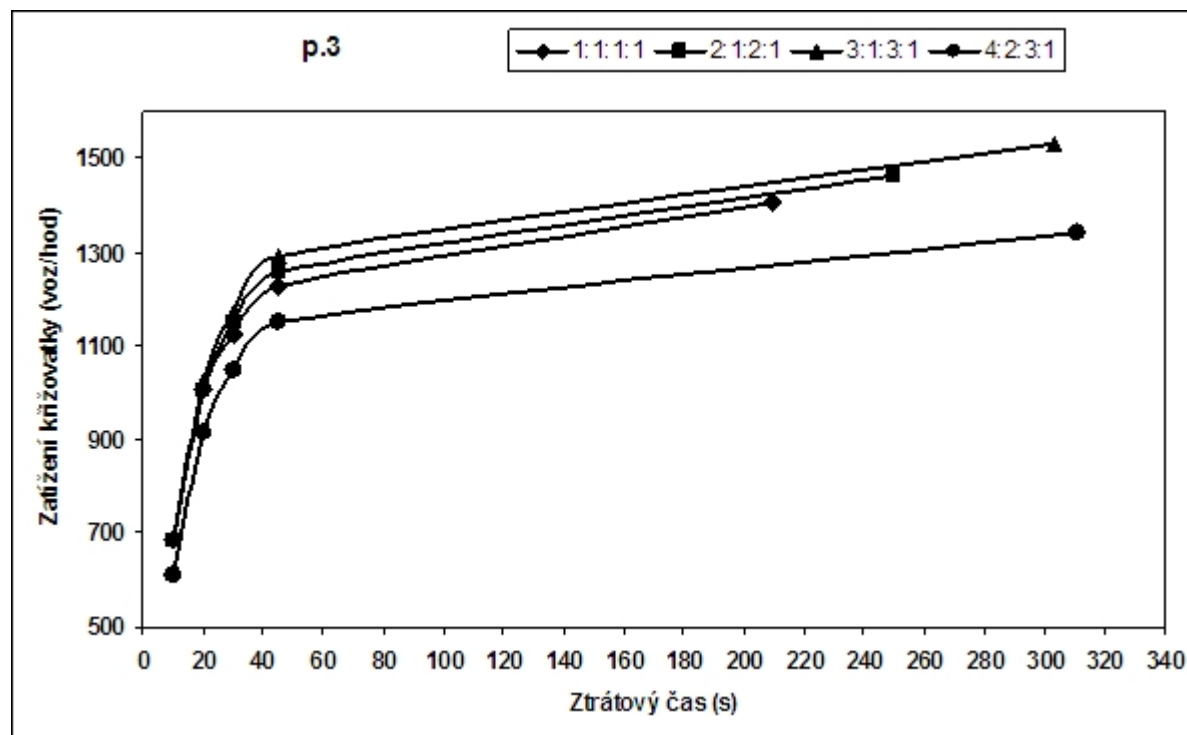
Zátěžové charakteristiky na dispozičním uspořádání p.3
