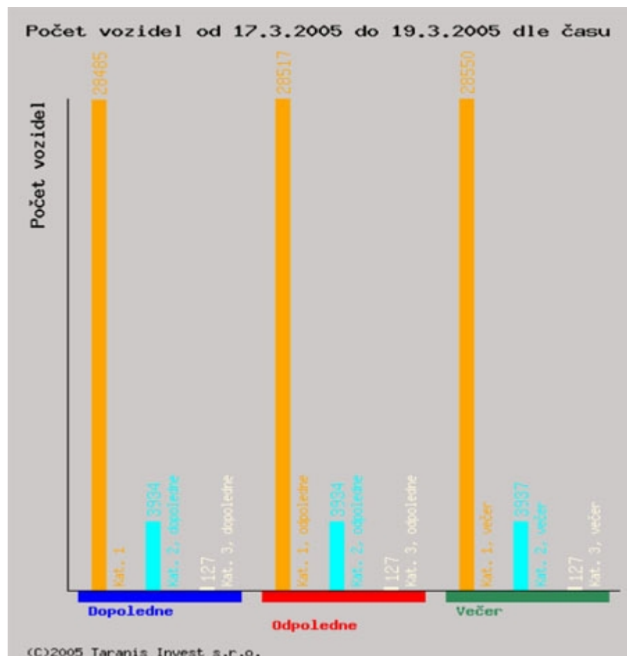
Obr. 3.7.1-1: Editace grafu
