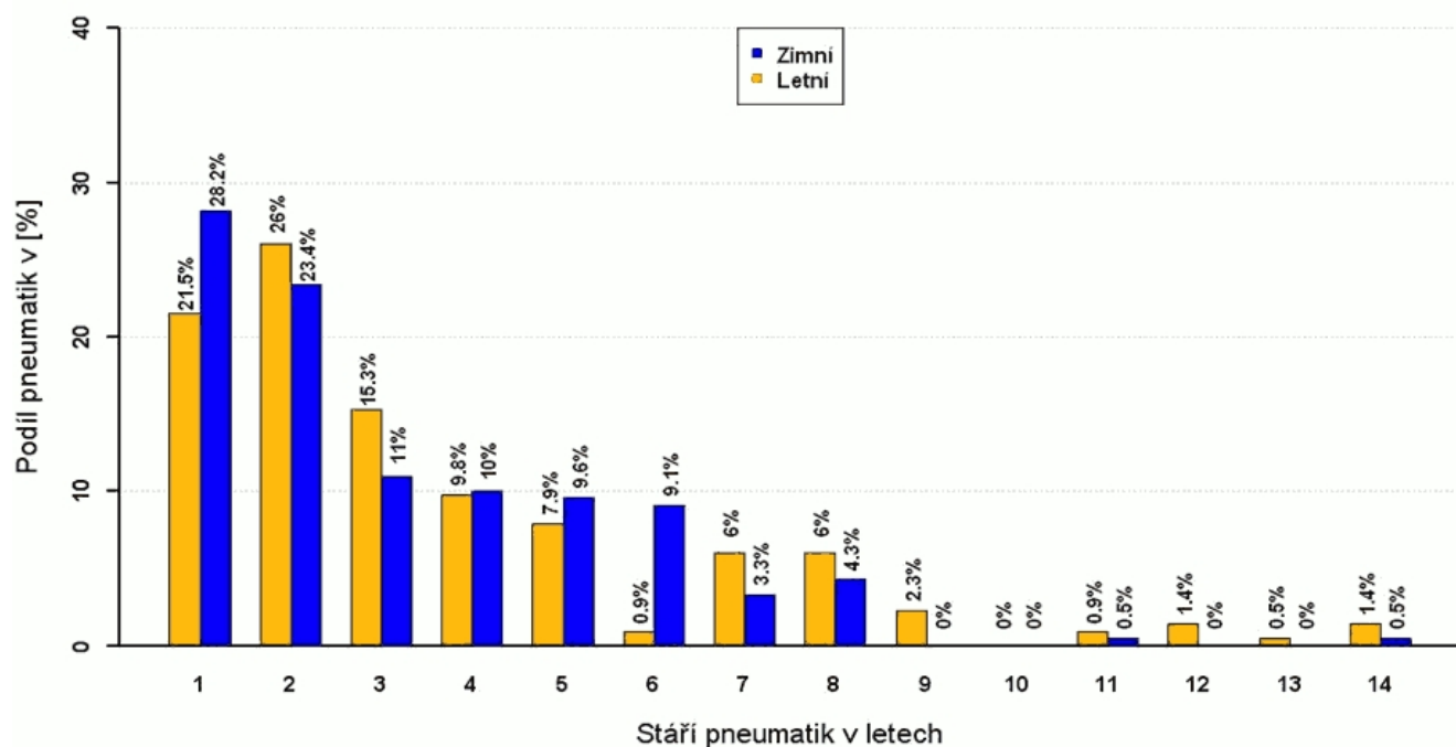
Graf 2.4 - Stáří pneumatik na osobních automobilech
