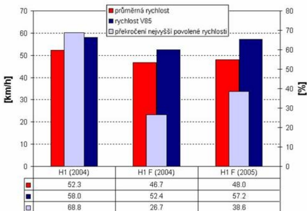
Obr. 7. Grafy a tabulky hodnot průměrné rychlosti, rychlosti V85 a procentuální četnosti překročení nejvyšší povolené rychlosti v profilu H1 na ulici Hranické (písmeno F označuje měření s figurínou)
