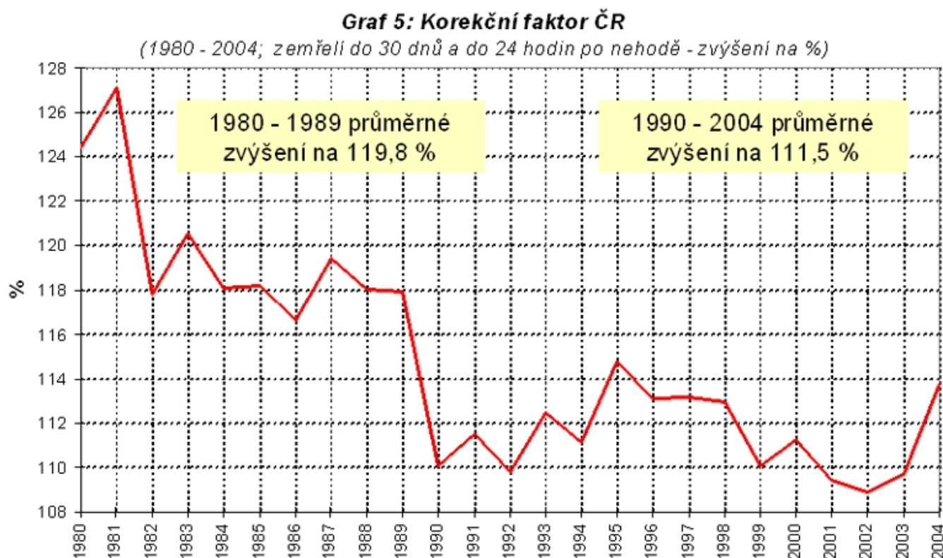
Graf 5: Korekční faktor ČR (1980 - 2004; zemřelí do 30 dnů a do 24 hodin po nehodě - zvýšení na %)
