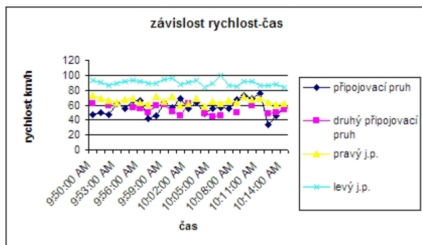
graf č. 1 (před změnou - typové schéma E1)
