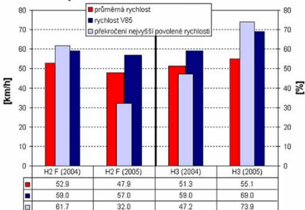
Obr. 8. Grafy a tabulky hodnot průměrné rychlosti, rychlosti V85 a procentuální četnosti překročení nejvyšší povolené rychlosti v profilech H2 a H3 na ulici Hranické (písmeno F označuje měření s figurínou)
