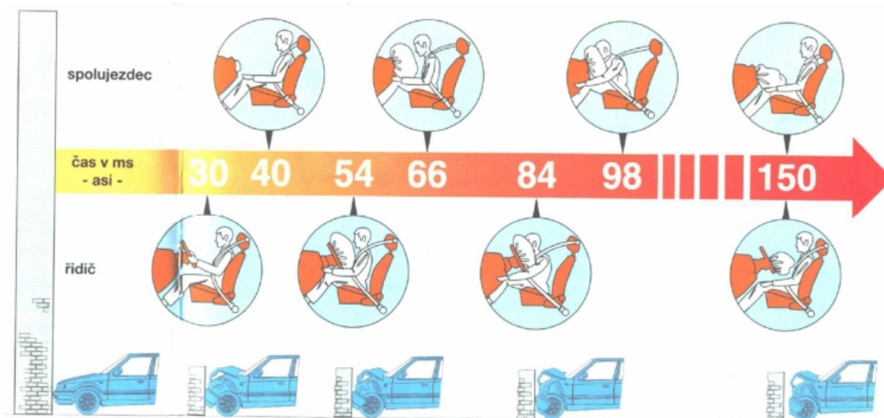
Obr. 1 - Průběh nafukování airbagu při nárazu [2]
